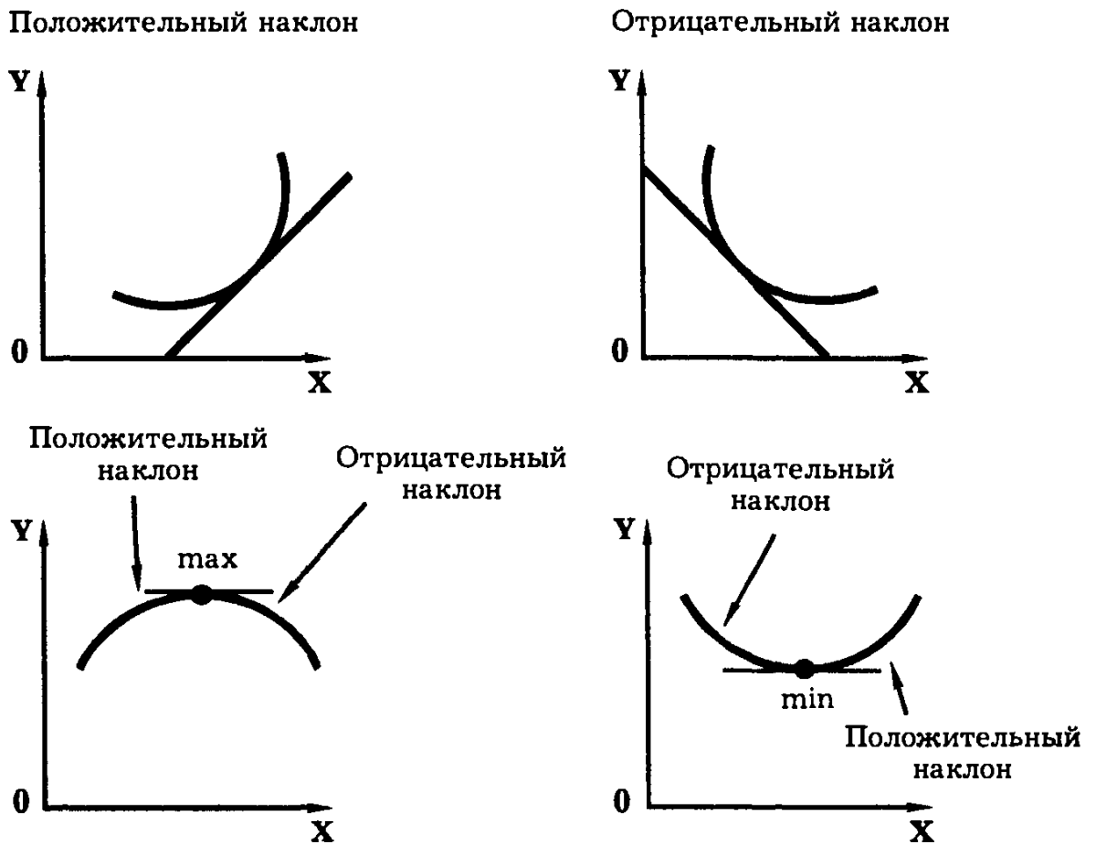
Рис. 1—11. Определение наклона кривых
